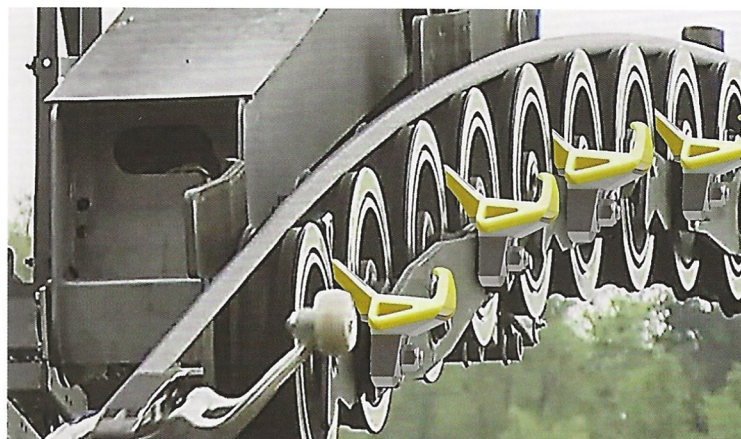
Die Artis Seilbahntechnik AG in Schlieren verfügt über ein breites Sortiment von Seilfängern für Skilifte sowie für Einseil-Umlaufbahnen.
